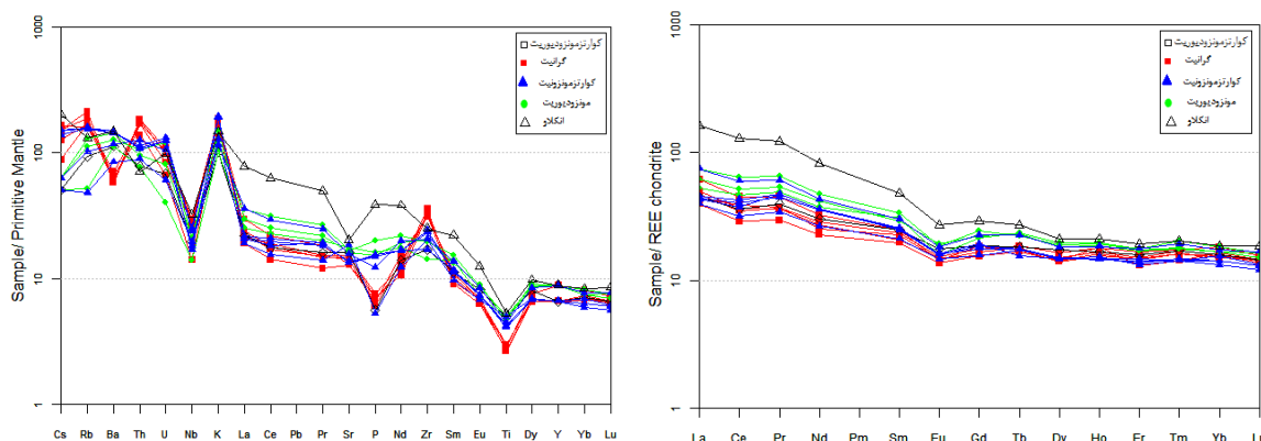
شکل ۱۳. نمودار عنکیوتی عناصر نادر خاکی سنگ‌های منطقه بررسی شده، که همه داده‌ها به کندریت [۱۸] عادی‌سازی شده‌اند، که تمامی داده‌ها به گوشته اولیه [۲۰] عادی سازی شده است
