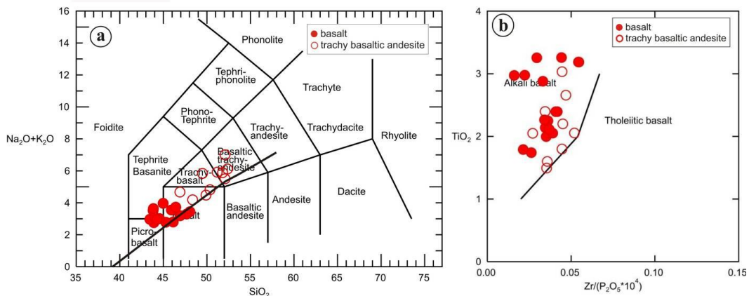
شکل ۳. (a) سنگ‌های آتشفشانی مرزن‌آباد در نمودار TAS [۱۸]، خط جداکننده سری‌های آلکان و کالک آلکان از
