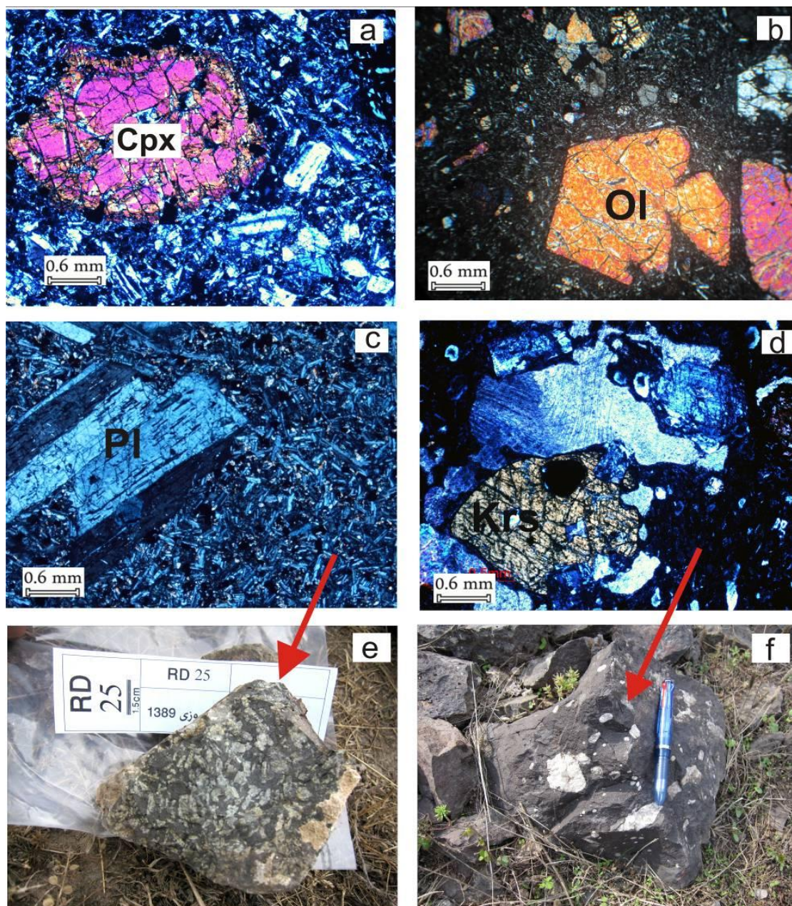
شکل ۲. تصاویر مقاطع نازک میکروسکوپی سنگ‌های بازیک جنوب مرزن‌آباد (به همراه a) کانی کلینوپیروکسن (Cpx) در نمونه بازالتی، b) کانی الیوین (Ol) در نمونه الیوین بازالتی، c) کانی پلاژیوکلاز (Pl) در نمونه تراکی آندزیت بازالت، d) کانی کرسوتیت (Krs) در نمونه تراکی آندزیت بازالت در حالت xpl، e) نمایی از نمونه دستی سنگ تراکی آندزیت بازالتی با ساخت پورفیری، f) نمایی از نمونه دستی سنگ تراکی آندزیت بازالتی با ساخت حفرهای علایم اختصاری نام کانی‌ها از [۱۲] اقتباس شده است.
