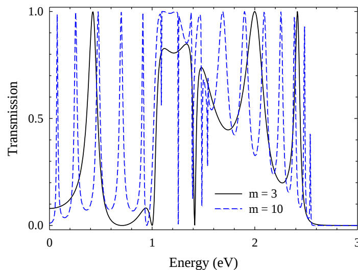
شکل ۲. نمودار ضریب عبور بر حسب انرژی الکترون ورودی برای دو نانونوار زیگززاگ با عرض n = 1 و طول‌های m = 3, 10
