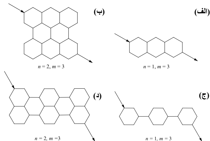
شکل ۱. چند مورد از نانونوارهای گرافن که از یک جایگاه در سمت چپ و از جایگاه متقابل در سمت راست به دو زنجیره اتمی متصل شده‌اند. (الف) و (ب) موارد زیگززاگ و (ج) و (د) موارد دسته صندلی را نشان می‌دهند. n و m به ترتیب نشان‌دهنده طول و عرض نانونوار هستند
