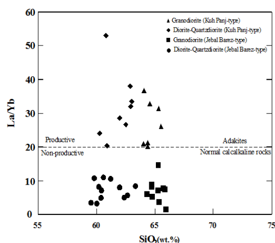
شکل ۸. تفکیک توده‌های نفوذی بارور از توده‌های نابارور در مقادیر \text{La/Yb} بیشتر از ۲۰
