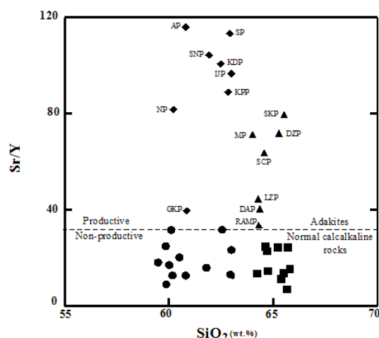
شکل ۵. تفکیک توده‌های نفوذی بارور (تیپ کوه پنج) از نابارور (تیپ جبال بارز) با استفاده از مقادیر نسبت Sr/Y در مقابل SiO_2
