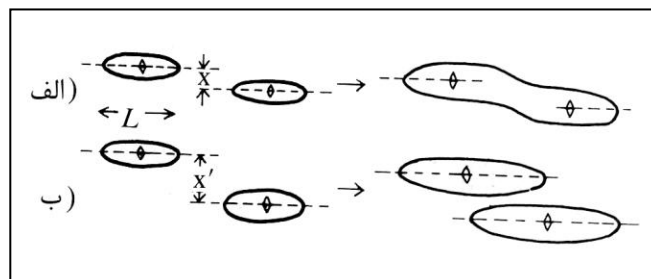
شکل ۱۱. الف) رشد و به‌هم آمیختن دو تاق‌دیس مجزا با جدایش کمتر از نصف طول موج ساختار، که باعث ایجاد خمیدگی محوری در تاق‌دیس حاصله شده است. ب) رشد دو تاق‌دیس مجزا با جدایش بیش از نصف طول موج ساختار، که باعث ایجاد دو تاق‌دیس هم‌پوشان، طویل و بدون خمیدگی محوری شده است [۲۰]
