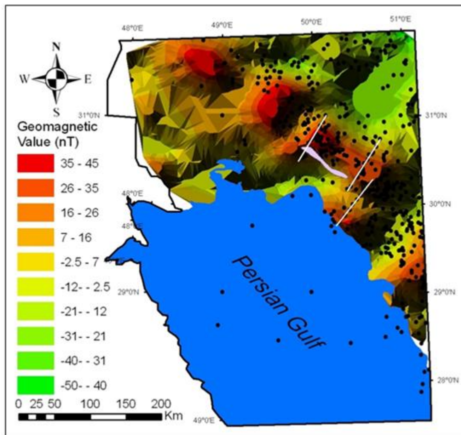
شکل ۹. انطباق تاقديس پازنان همراه با کانون‌های لرزه‌ای بر روی نقشه انطباق‌یافته ژئومغناطیس پی‌سنگ [۴] در فروافتادگی دزفول و نواحی اطراف (با توجه به کانون خطی زلزله‌ها خطوط سفید گسل‌های پی‌سنگی احتمالی یا بلندای‌های احتمالی قدیمی را نشان می‌دهد)
