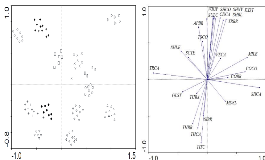
شکل ۱. شکل حاصل از PCA با استفاده از داده‌های کیفی. شکل سمت چپ توزیع نمونه‌ها و شکل سمت راست توزیع صفات را بر روی دو محور نمایش می‌دهد. \triangle گونه S. aethiopsis ، \times گونه S. chloroleuca ، \diamond گونه S. nemorosa ، \blacklozenge گونه S. scalrea ، \blacklozenge گونه S. ceratophylla ، \blacklozenge گونه S. shariffi ، \nabla گونه S. reuterana ، + گونه S. macrosiphon ، \blacklozenge گونه S. leriifolia ، \square گونه S. atropatana ، \square گونه S. virgata ، \square گونه S. chorassanica ، \blacklozenge گونه S. spinosa (PC1 = %71)
