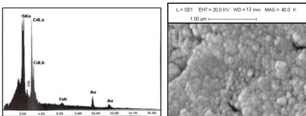
شکل ۴. تصویر SEM و EDX نانوذرات CdS:Fe(4%) ([TG]= ۰/۰۹ M).
