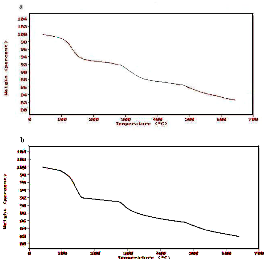
شکل ۱۱. TGA نمونه، (a) با Rate = ۵ و (b) با Rate = ۱۰
