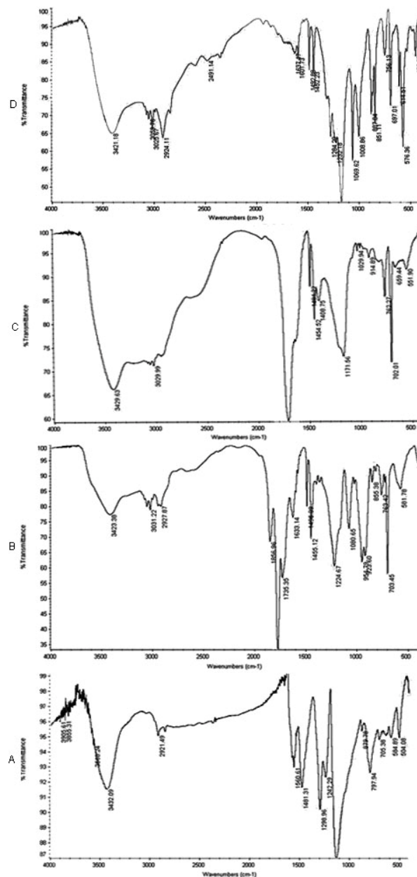
شکل ۴. طیف‌های IR مربوط به PSS (D)، PSMA (B)، PANI/HCl (A)، PSSMAC (C)
