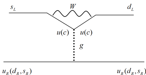
شکل ۱. نمودار فاینمن مربوط به عملگرهای پنگوئن
