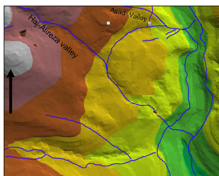
شکل ۴. مدل TIN سال ۴۳ محدوده توده لغزشی
