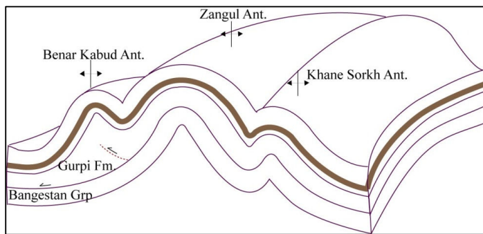
شکل ۴. بلوک دیاگرامی از تاقديس‌های فرعی در پهلوهای تاقديس زنگول
