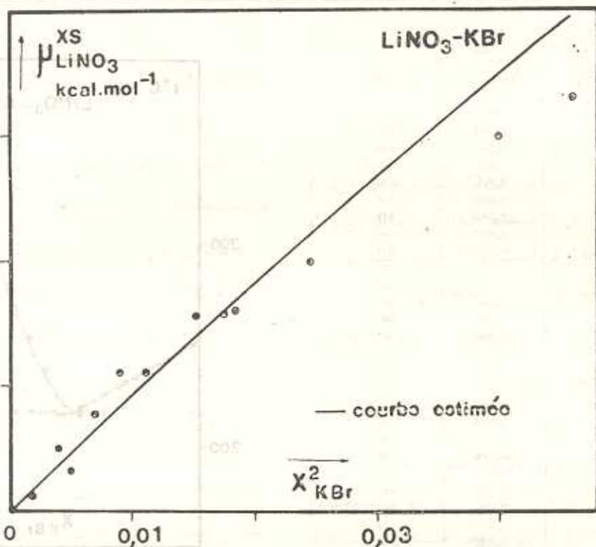
شکل ۲- تغییر پتانسیل شیمیایی نیترات لیتیم بر حسب غلظت
