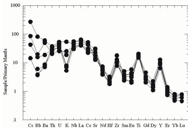
شکل ۷. نمودار چندعنصری نرمالیز شده با گوشته اولیه [۷]
