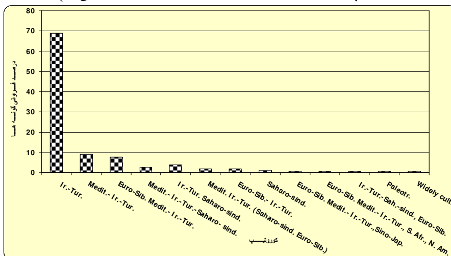
شکل ۵. درصد فراوانی پراکنش جغرافیایی گونه‌های گیاهی ارتفاعات کلات_ زیرجان گناباد (Euro-Sib. Ir.-Tur.، Meditrane، Euro-Sib.، Saharo-sind.، Sino-Jap.، S. Afr.، N. Am.، Paleotr.، به ترتیب بیان‌گر ایرانی-تورانی، مدیترانه‌ای، اروپا-سیبری، صحرا-سندی، سینو-ژاپنی، آفریقای جنوبی، آمریکای شمالی، پالئوتروپیک است)
