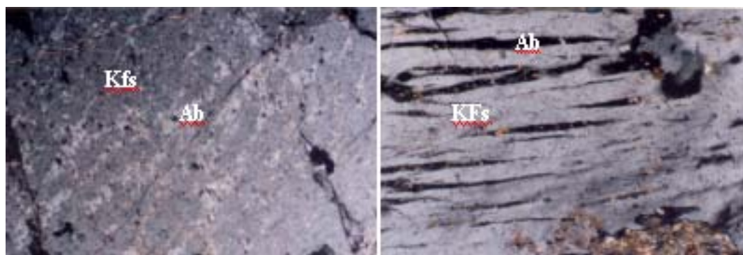
شکل ۹. هم‌رشدی‌های پرتیتی (سرد شدن و اختلاط ناپذیری) در گرانیتهای شمال موته (×100.XPL). فلدسپات پتاسیک = Kfs و آلبیت = Ab
