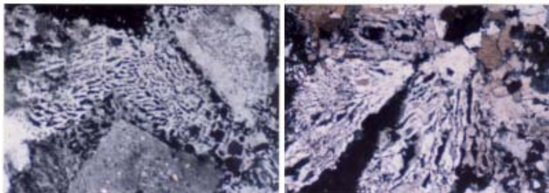
شکل ۷. نمایش بافت گرانوفیر در گرانیتهای دره ریز آب در شمال شرق گلپایگان (×100.XPL)
