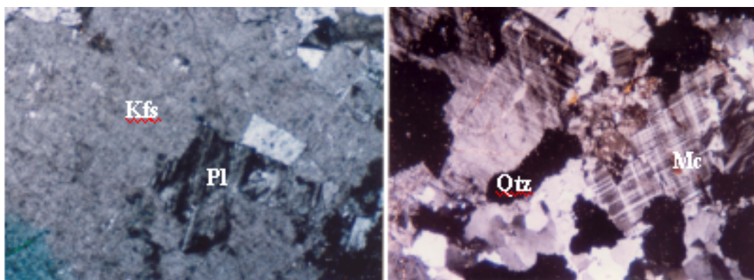
شکل ۵. تصویر بافت بوئی کلبیتی که در آن فلدسپات پتاسیک پلاژیوکلاز را در بر گرفته است (×100.XPL) فلدسپات پتاسیک = Kfs و پلاژیوکلاز = Pl
