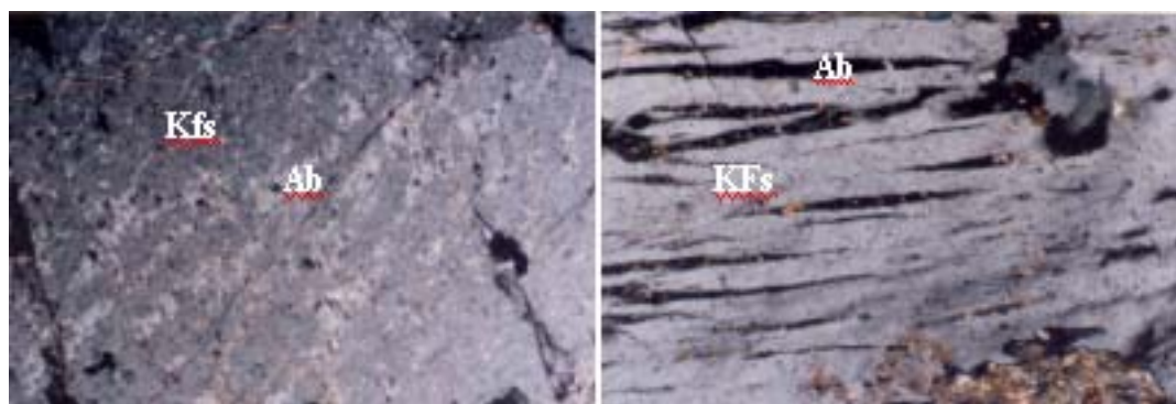
شکل ۹. هم‌رشدی‌های پرتیتی (سرد شدن و اختلاط ناپذیری) در گرانیت‌های شمال موته ( \times 100.XPL ). فلدسپات پتاسیک = Kfs و آلبيت = Ab
