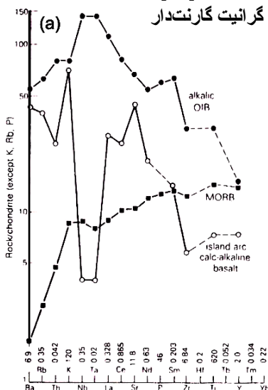
شکل ۱۱- (a) نمودار عنکبوتی برای MORB، OIB و جزایر قوسی (IAB) نرمالیزه شده براساس تامپسون و همکاران (۱۹۸۲) [اقتباس از ویلسون، ۱۹۸۹] (b) نمودار عنکبوتی دیوریت‌های بائه نرمالیزه شده براساس تامپسون و همکاران (۱۹۸۲)
