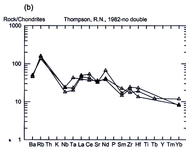
شکل ۱۱- (a) نمودار عنکبوتی برای MORB، OIB و جزایر قوسی (IAB) نرمالیزه شده براساس تامپسون و همکاران (۱۹۸۲) [اقتباس از ویلسون، ۱۹۸۹] (b) نمودار عنکبوتی دیوریت‌های بائه نرمالیزه شده براساس تامپسون و همکاران (۱۹۸۲)
