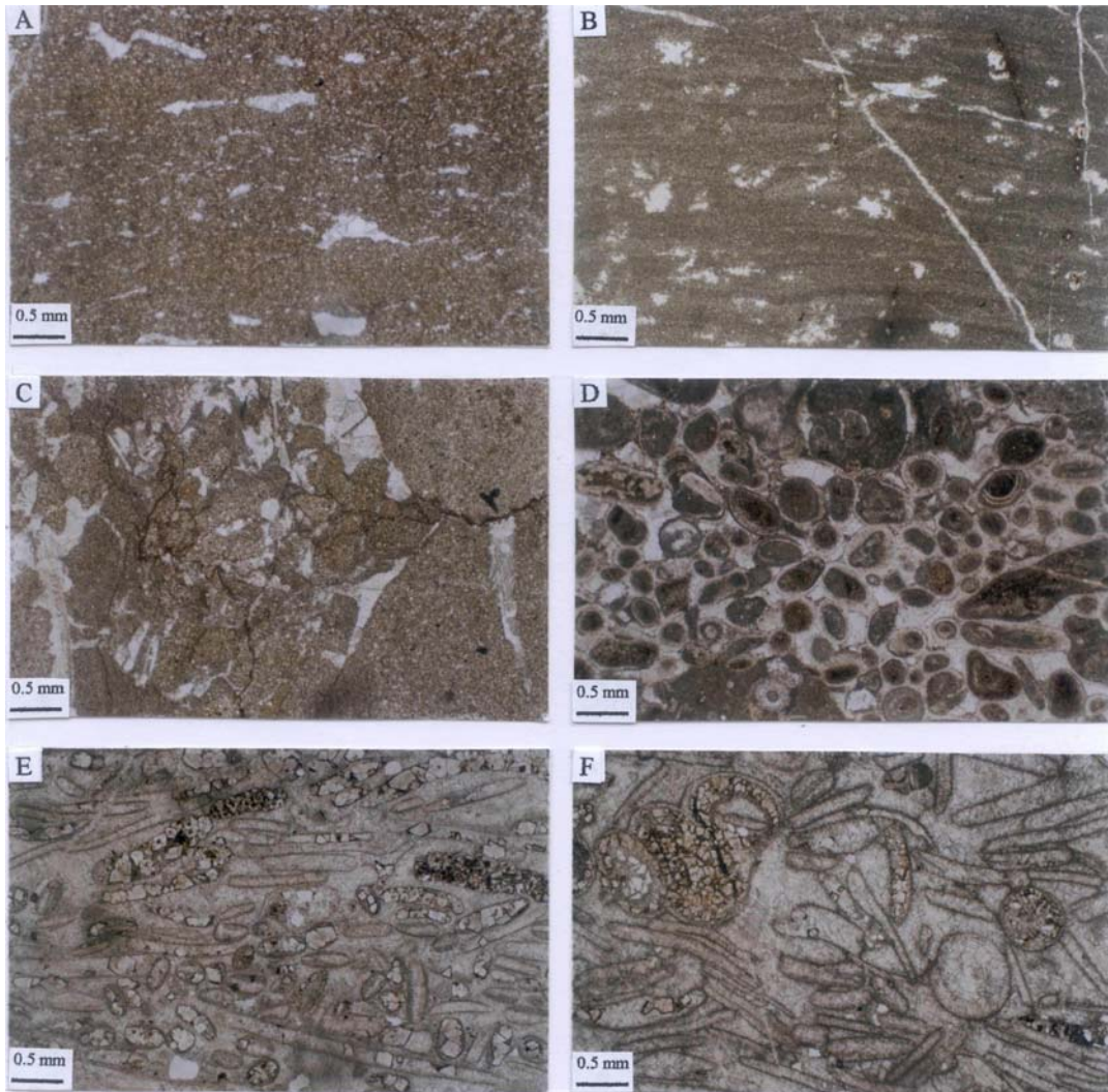
شکل ۴- A- دولومدستون با فابریک چشم پرنده‌ای مربوط به رخساره C ، مقطع توسط الیزارین قرمز رنگ آمیزی شده است (نمونه برش گذار سرخ) B- دولومدستون لامینه‌دار با فابریک چشم پرنده‌ای و قالب‌های دروغین ژپس و انیدریت در رخساره C، مقطع توسط الیزارین قرمز رنگ آمیزی شده است (نمونه از برش اسلام‌آباد) C- گرینستون اینتراکلاستی از رخساره طوفانی کریناته، در این تصویر، اینترکلاست‌های میکریتی بوده‌اند و فابریک سیمان از نوع هم بعد است. بالای مقطع به سمت چپ عکس است بنابراین ساختمان رسوبی از نوع لایه‌بندی تدریجی نیز در اینجا مشاهده می‌گردد (نمونه از برش گذار سرخ) D- گرینستون الیدی اینتراکلاستی مربوط به رخساره طوفانی کریناته. الیدها دارای فابریک‌های شعاعی و متحد‌المرکز هستند. فابریک سیمان نیز غالباً از نوع هم بعد است (نمونه از برش گذار سرخ) E- گرینستون بیوکلاستی الیدی از رخساره طوفانی کریناته. الیدها دارای فابریک متحد‌المرکز بوده و دوکفه‌ای‌ها نیز توسط کلسیت اسپاری پر شده‌اند. فابریک‌های سیمان از نوع دروزی موزائیکی و هم قعد هستند بلورهای اتومورف دولومیت نیز به وضوح دیده می‌شوند. برخی از آنها حالت زونه مانند نیز دارند (نمونه از برش گذار گچال) F- گرینستون بیوکلاستی در رخساره طوفانی کریناته. بیوکلاست‌ها شامل دوکفه‌ای و شکم‌پایا دیواره اسپاریتی هستند. فابریک‌های سیمان از نوع هم بعد و دروزی موزائیکی‌اند جانشینی بلورهای اتومورف دولومیت در برخی از آوکه‌ها دیده می‌شوند (نمونه از برش گذار گچال)
