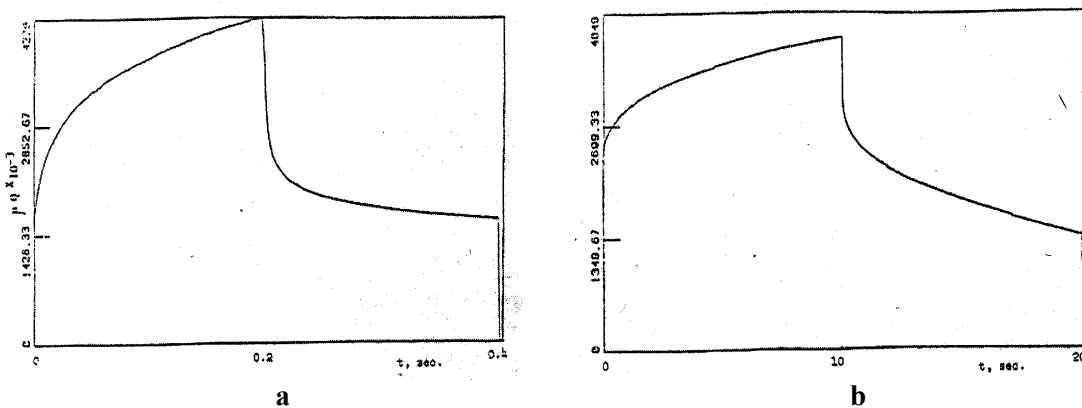
شکل ۴- (a) منحنی کروماتوگرافی الکترودهای نازک طلا 300 \text{ \AA} در الکترولیت 0.1 \text{ mol LiClO}_4 ، تغییرات پتانسیل از 0.5 به 0.35 ولت نسبت به SCE (b) منحنی کروماتوگرافی الکترودهای نازک ( 1000 \text{ \AA} ZnPC) در الکترولیت 0.1 \text{ mol LiClO}_4 ، تغییرات پتانسیل از 0.5 به 0.35 ولت نسبت به SCE
