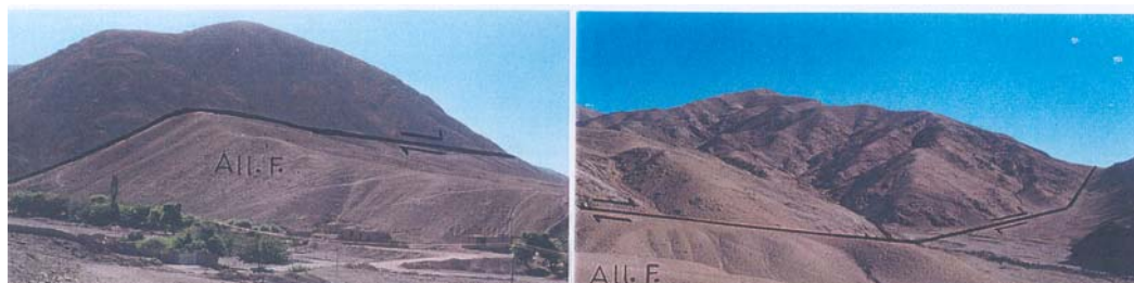
شکل ۸- ب) مخروط افکنه نزدیک و در مجاور قطعه خانوک گسل کوهبنان، Ail.F: مخروط افکنه ج) مخروط افکنه نزدیک و در مجاور قطعه ریگ‌آباد گسل کوهبنان با نیمرخ گوه‌ای، حداکثر ضخامت مخروط افکنه در مجاورت پیشانی گسلی کوهستان، Ail.F: مخروط افکنه
