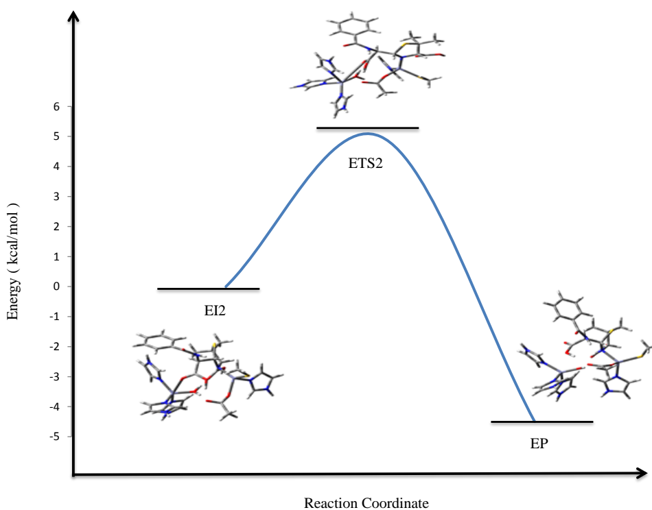
شکل ۱۴. نمودارهای انرژی پتانسیل کمپلکس مدل آنزیم CcrA با پنی‌سیلین مسیر اول واکنش، حمله نوکلئوفیلی گروه هیدروکسید پل به سویسترا (نمودار اول) و مسیر دوم واکنش، پروتونه شدن گروه آمین (نمودار دوم) هستند
