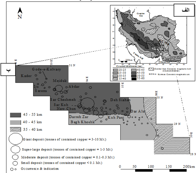
شکل ۲. الف) نقشه ساده شده ضخامت پوسته در گستره ایران بر پایه نقشه عمق امروزی موهو [۴۸] (ب) نقشه تعبیرات ضخامت پوسته قاره‌ای در سراسر کمان ماگمایی سنوزوییک کرمان و تمرکز کانسارهای اصلی مس پورفیری در بخش‌های شمال غربی کمان که منطبق بر حداکثر ضخامت پوسته است [۱۷]
