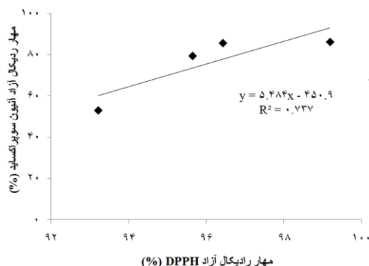
شکل ۲. رابطه میان فعالیت آنتی‌اکسیدانی به روش مهار رادیکال آزاد DPPH و فعالیت مهار رادیکال آزاد آنیون سوپراکساید در عصاره گونه سالویا اتیوپیسی
