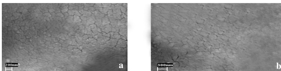
شکل ۷. تصاویر میکروسکوپ الکترونی از تزئینات سطح آگزین دانه‌های گرده با بزرگ‌نمایی ۲ و ۵ ماکرومتر (a) اوتریکولاریا استرالیس و (b) اوتریکولاریا مینور
