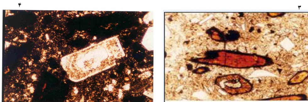
شکل ۳. بلورهای هورنبلند با حاشیه سوخته در آندزیت‌های منطقه آشتیان (5X10 XPL)
